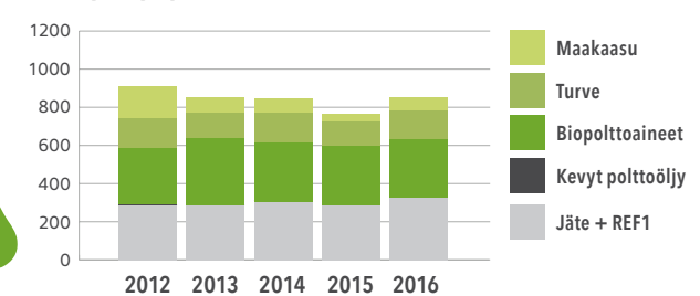
Käytetyt polttoaineet, GWh
